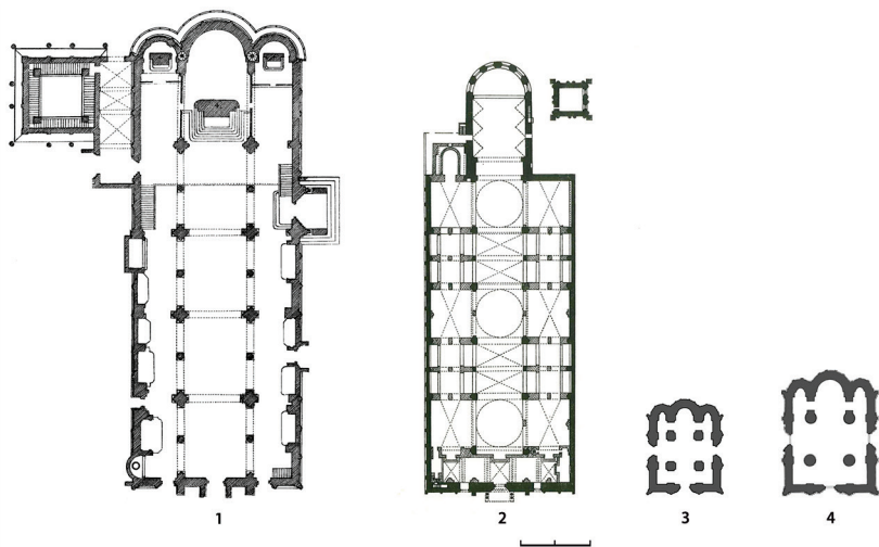
Рис. 1. Сравнение планов: 1 — собор в Модене; 2 — собор в Ферраре; 3 — церковь Покрова на Нерли; 4 — церковь Рождества Богородицы в Боголюбове
